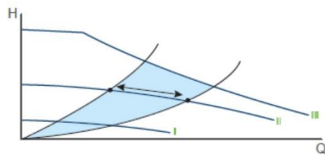
Konstantní křivka/křivka otáček
