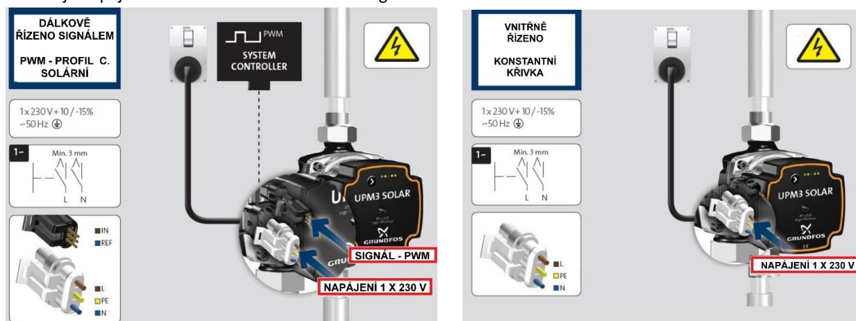
Zapojení při řízení signálem PWM
