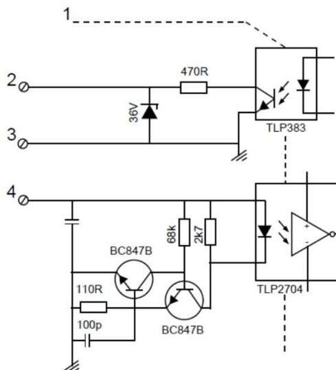
Schematický náčrt, rozhraní
